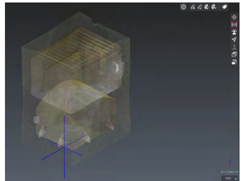
Fig. 16- Fase 1: nube de puntos parcial para el estudio de la bóveda de PBaja (torre suroeste). Ubicación del pto de ref.0.00. (Autores)
