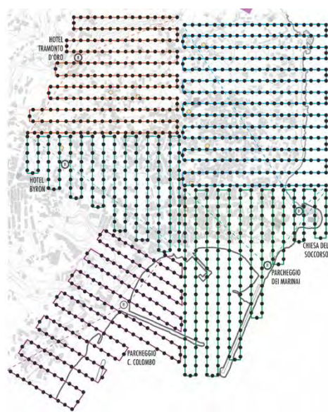
Fig. 4- Piano di volo su Forio d'Ischia (Patryk Rynkowski, 2024)
