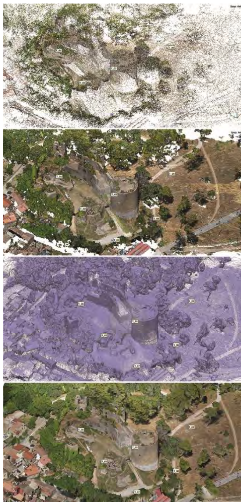
Fig. 9- Dall'alto verso il basso: nuvola di punti sparsa; nuvola di punti densa; modello mesh; modello mesh texturizzato (elaborazione grafica di Domenico Iovane & Rosina Iaderosa, luglio 2025)
