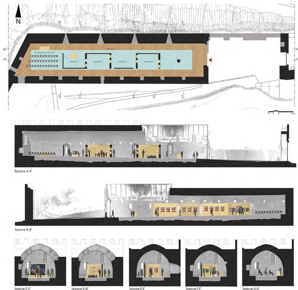
Fig. 4- Progetto di musealizzazione delle scuderie del castello (elaborazione grafica degli autori, 2025)
