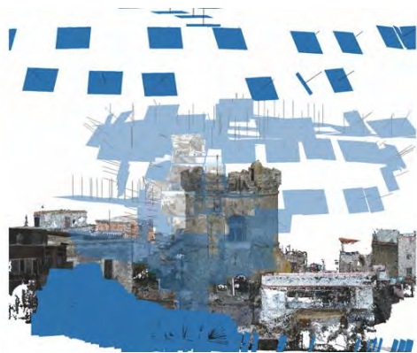
Fig. 10- Torrione, nuvola densa con allineamento foto aeree e terrestri (Patrik Rynkowski, 2024)
