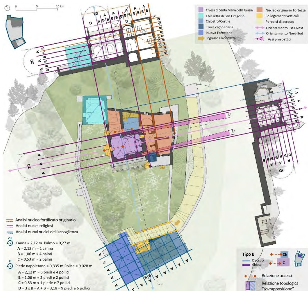
Fig. 4- Analisi grafico-metrica-topologica del complesso monastico/fortificato (a cura degli autori)
