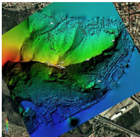
Fig. 11- Vista del MDE generado en el proceso fotogramétrico con Metashape Profesional de Agisoft (Autores)
