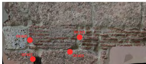
Fig. 2- Localizzazione dei quattro campioni raccolti sulla facciata Sud-Est della torre di via dei Montanini n.16 – quota 2,40 ca. dal piano strada (elaborazione grafica degli autori, 2025)
