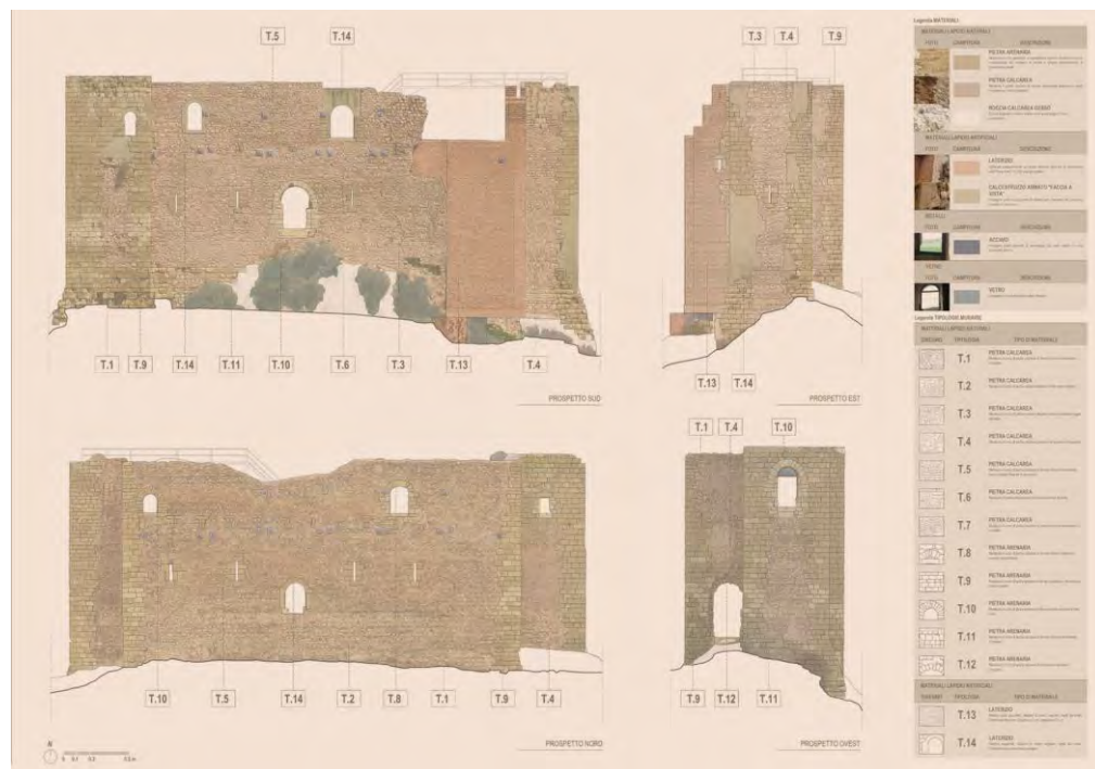
Fig. 3- Caratterizzazione materica e tipologico-costruttiva dei fronti (autori)
