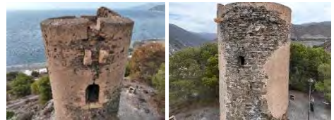
Figs. 4a, 4b- Imagen de caras norte (a) y sur (b) de torre Melicena con grieta vertical que se prolonga por el lateral Este
