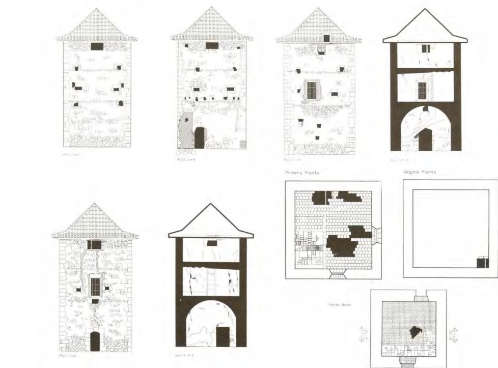
Fig. 8- Planimetría y alzado de la torre de Tadeo (Melchor, Benedito y Ferrer, 2001)
