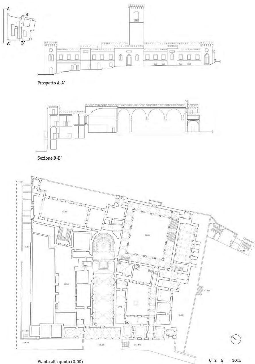
Fig. 4- Castello Guglielmi, ipotesi ricostruttiva, pianta, prospetto e sezione (elaborazione grafica di Chiara Spipoli, 2025)
