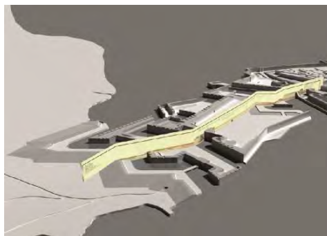
Fig. 5- Il modello digitale tridimensionale raffigurante lo stato delle fortificazioni al 1842, realizzato a partire dalla pianta e dalle sezioni della Real Piazza (a cura dell'autrice)
