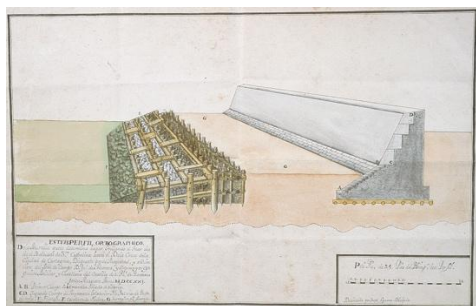
Fig. 2- Plano de 1721 que muestra la sección de la muralla a construir y la escollera sumergida. (A) y (B) son el primer cuerpo de la muralla asentado en bloques de sillería, (C) y (D) son el segundo cuerpo hecho de argamasa con paramentos de sillería, (E) son los pilotes, (F) es la escollera de piedra y (G) es el terraplén para fuerza (España, Ministerio de Cultura y Deporte, Archivo General de Indias, Panamá, 124)
