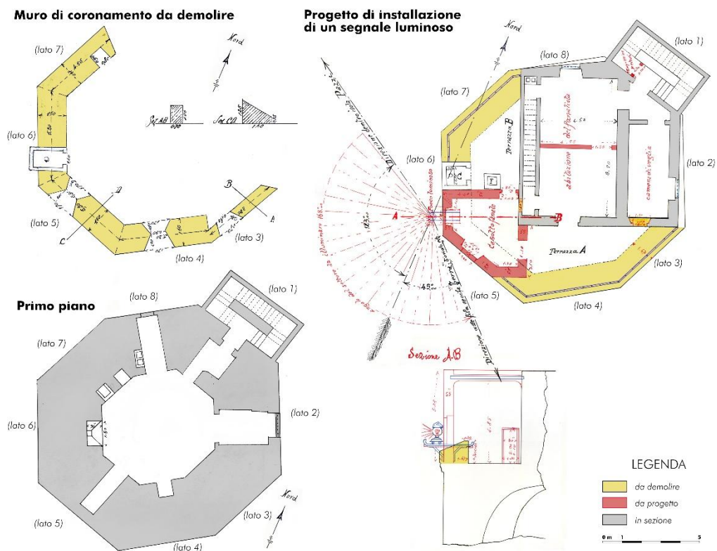
Fig. 3- Torre San Giovanni, Ugento (Le): tavole tecniche inerenti il progetto del 1931 per l'installazione di un segnale luminoso (Archivio di Stato di Lecce, rielaborazione grafica a cura degli autori)
