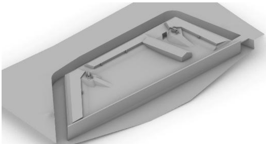
Fig. 5– Ricostruzione 3D della Batteria progettata, ma mai realizzata dell’Annunziata
