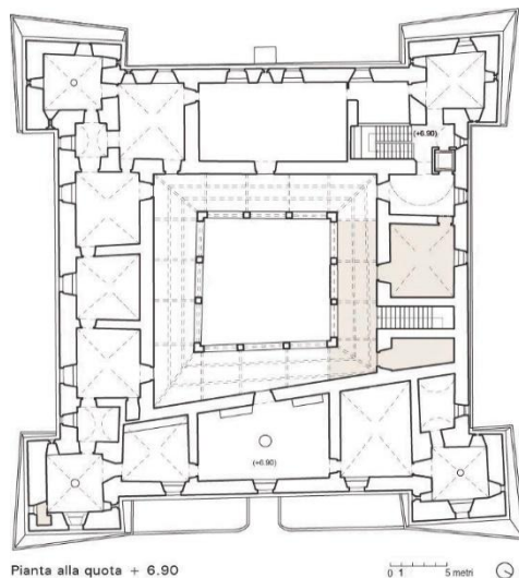
Fig. 8- Rilievo architettonico della Castellina a Norcia, pianta alla quota + 6,90 m (elaborazione grafica di Serena Pallotti, 2025)
