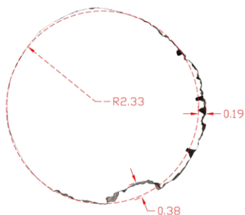
Fig. 8- Sección en planta de torre. Se comprueba la deformación excentrica hacia el este y la pérdida de material del muro
