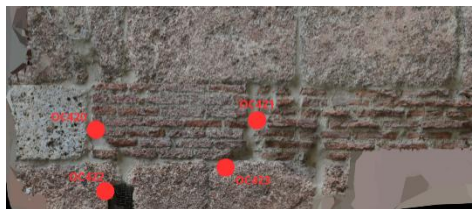
Fig. 2- Localizzazione dei quattro campioni raccolti sulla facciata Sud-Est della torre di via dei Montanini n.16 – quota 2,40 ca. dal piano strada (elaborazione grafica degli autori, 2025)
