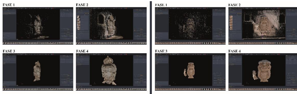
Fig. 7- Processo di restituzione grafica degli Stemmi mediante il software 3DF Zephyr. A sinistra lo Stemma Imperiale di Carlo II d'Asburgo; a destra quello del Viceré Don Claudio Lamoral, principe di Ligne (a cura dell'autrice)
