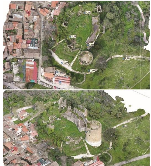
Fig. 8- Visualizzazione sul modello texturizzato dei GCP (elaborazione grafica di Domenico Iovane & Rosina Iaderosa, aprile 2025)
