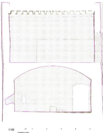
Fig. 19- Fase 4: Elección de la sección generada por plano YZ por pto de ref. 0.00 y su delineación en Autocad. Sección escalada y utilizada para su análisis con estática gráfica con la geometría real de sus muros y trazo de la bóveda. (Autores)
