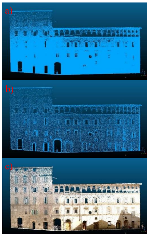
Fig. 4a-b-c- Vista ortocorretta del prospetto su via Cecco Angiolieri: a) nuvola di punti completa; b) nuvola di punti sub-campionata a 0.03 cm; c) nuvola di punti con texture (elaborazione grafica degli autori, 2025)
