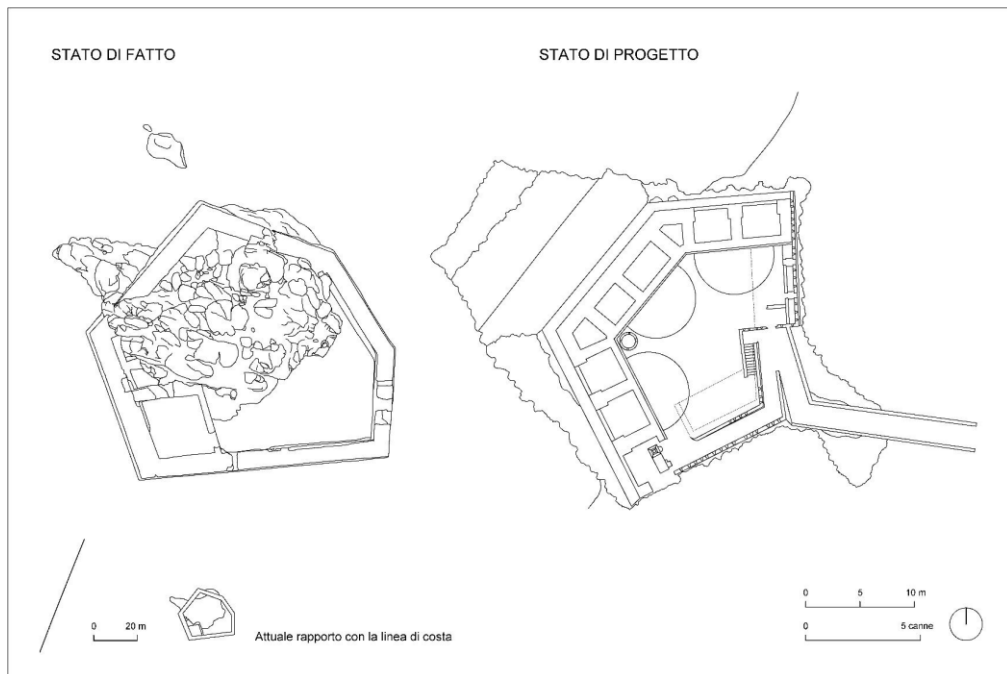
Fig. 6- Confronto tra lo stato di progetto e lo stato di fatto (Elaborazione F. Stilo)
