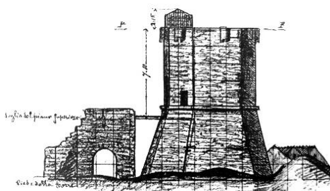
Fig. 2- Torre San Giovanni nella marina di Ugento (Le): prospetto quotato del 1870 (Cazzato, Politano: 2001, p. 126)
