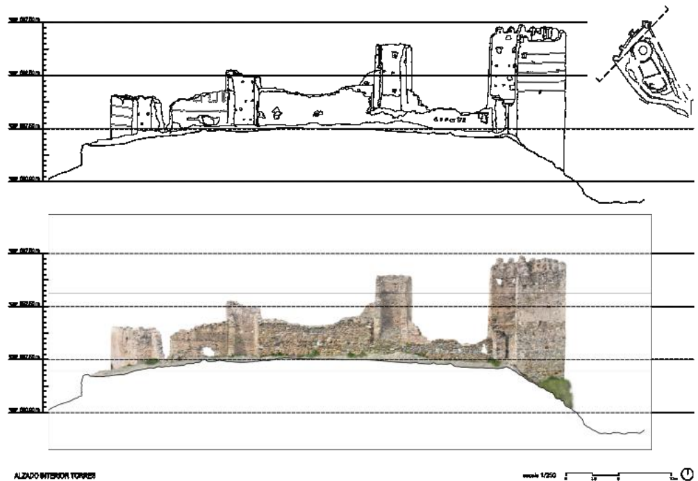
Fig. 8- Alzado interior noroeste del castillo de Alcudia de Veo (elaboración gráfica por Ana Pérez-Vila, Teresa Gil-Piqueras & Pablo Rodríguez-Navarro, 2025)
