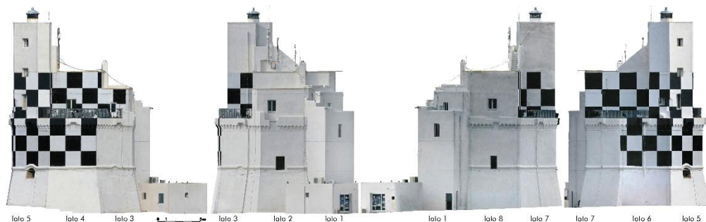
Fig. 5- Faro di Torre San Giovanni, Ugento (Le). Rilievo fotogrammetrico: prospetti esterni
