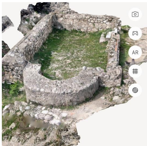
Fig. 7- Rilievo di dettaglio con metodologia LiDAR mediante app Polycam: resti della chiesa dedicata a Skanderbeg (elaborazioni e restituzione grafica di Angelo De Cicco)
