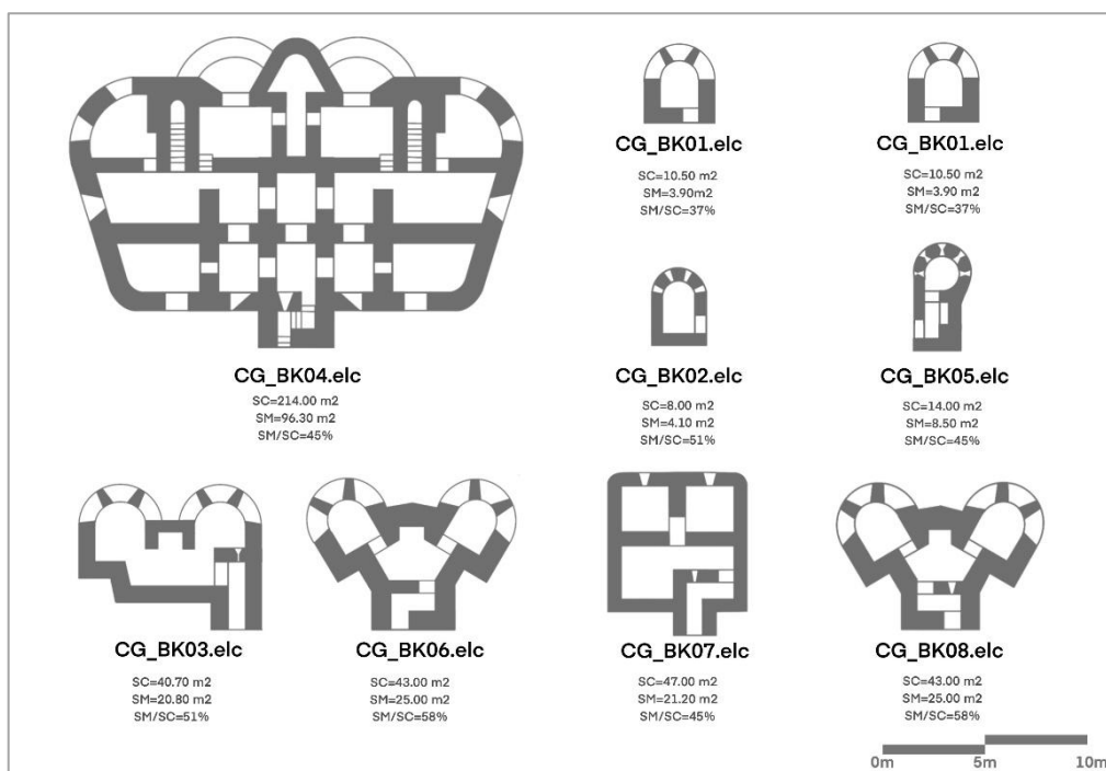
Fig. 2- Inventario de las plantas de los 8 búnkeres del Clot de Galvany (CG) numeradas de este a oeste, desde el mar hacia tierra, y que nombramos con el acrónimo BK (búnker) seguido de su numeración: desde el CG-BK01.elc, cerca de la playa de Carabassí, hasta el CG-BK08.elc, al otro lado de la carretera nacional, destacando el CG-BK04.elc por ser el mayor (214.00m 2 ), presentar dos niveles y situarse en la pequeña isla de la laguna. A poniente de la carretera hay un par de trincheras excavadas en lo alto de una loma del Cabeçó y, hacia el noreste, se sitúan tres baterías anticarro BC de otra zona (fuente: autores)
