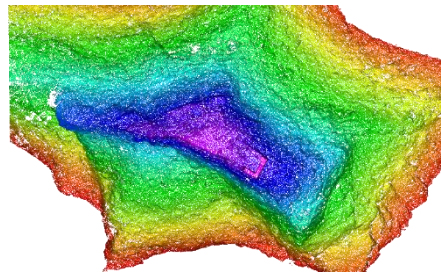
Fig. 20- Modelo 3d de nube de puntos con escala de elevaciones a partir del proceso fotogramétrico con Metashape de Agisoft. Visualizado con Recap Pro de Autodesk. (Autores)
