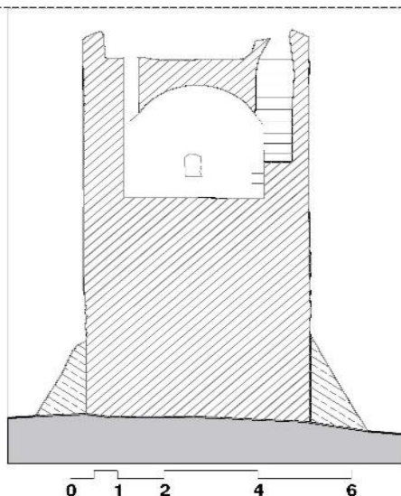
Fig. 9- Sección de la torre de Melicena
