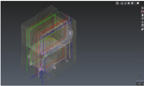
Fig. 18- Fase 3: Generación de secciones a la generatriz de la bóveda a estudio para su elección óptima. (Autores)
