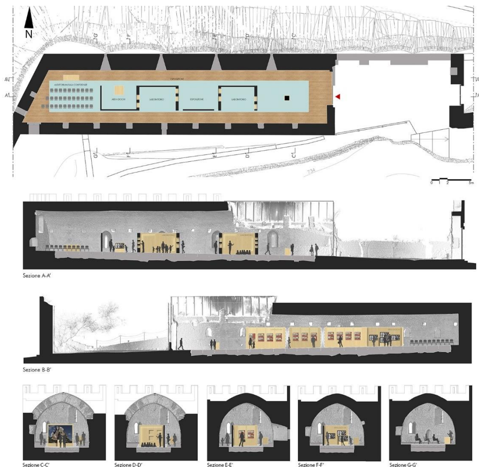
Fig. 4- Progetto di musealizzazione delle scuderie del castello (elaborazione grafica degli autori, 2025)
