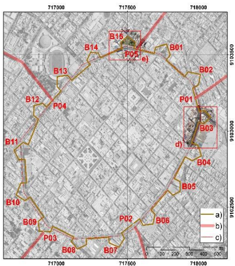
Fig. 6- Reconstrucción digital del trazado de la muralla de Trujillo. a) trazado de la muralla, b) caminos virreinales, c) centro histórico, d) cortina de la avenida España y el resto del baluarte del Señor Obispo, e) baluarte de Don Juan de Herrera y Valverde
