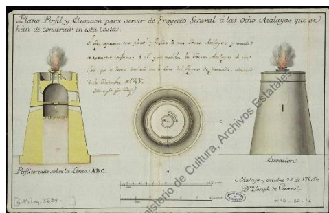
Fig. 1- Plano de planta, alzado y sección proyecto torres atalayas en s XVIII (Archivo Estatal de Simancas)
