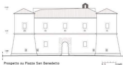
Fig. 9- Rilievo architettonico della Castellina a Norcia, prospetto su piazza San Benedetto (elaborazione grafica di Serena Pallotti, 2025)
