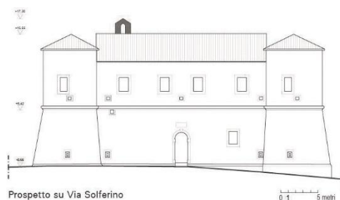
Fig. 10- Rilievo architettonico della Castellina a Norcia, prospetto su via Solferino (elaborazione grafica di Serena Pallotti, 2025)
