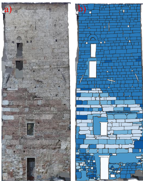
Fig. 4 a-b- a) Ortoproiezione della facciata Sud-Est della torre: b) mappatura litologica (elaborazione grafica degli autori, 2025)
