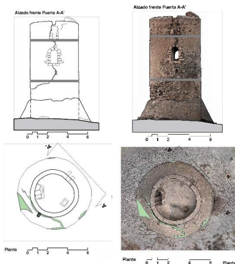
Fig. 10- Propuestas de consolidación de la torre de Melicena mediante colocación de dos cinchas de acero que abrazan y restauración de huecos mediante mortero de cal con mampuestos
