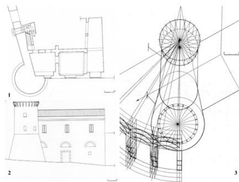
Fig. 8. Disegni analogici della torre di Sessa Aurunca (CE): 1) pianta, 2) prospetto, 3) assonometria (elaborazione grafica di Michele Sabatino)
