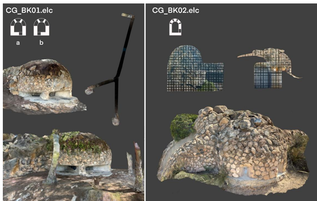
Fig. 3- Levantamientos fotogramétricos de los búnkeres BK01.elc y BK02.elc que se basan en unidades de búnker de un solo seno. El CG-BK01 (izq.) está compuesto por dos pequeños búnkeres a los que se accede por una galería posterior excavada, cada uno equipado con mesa para ametralladora barriendo una zona de 180° del campo de tiro. El CG-BK02 (dch.), más que un búnker es una casamata como puesto de vigilancia y control sobre el destacamento y el mar, con aspilleras para fusiles (fuente: G. Sanna, 2025)
