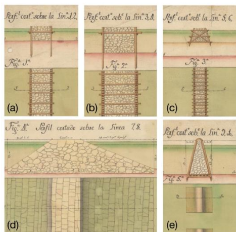
Fig. 6- Detalles del Plano general de la plaza de Cartagena de Indias, por Antonio de Arévalo (1769 plano 2), donde (a) es la propuesta de Josep de Herrera, (b) la de Carlos Desnaux, (c) la de Ignacio de Sala, (d) la de Manuel Hernández y (e) la de Lorenzo de Solís ( España, Ministerio de Defensa, Instituto de Historia y Cultura Militar, Archivo General Militar de Madrid. Sig. COL 16-05 )
