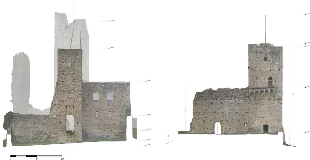
Fig. 6- Prospetti con inserimento dei fotopiani del fronte sud/est della Postierla (sinistra) e fronte nord/ovest della torre delle Prigioni (destra) (Fantoni, 2025)
