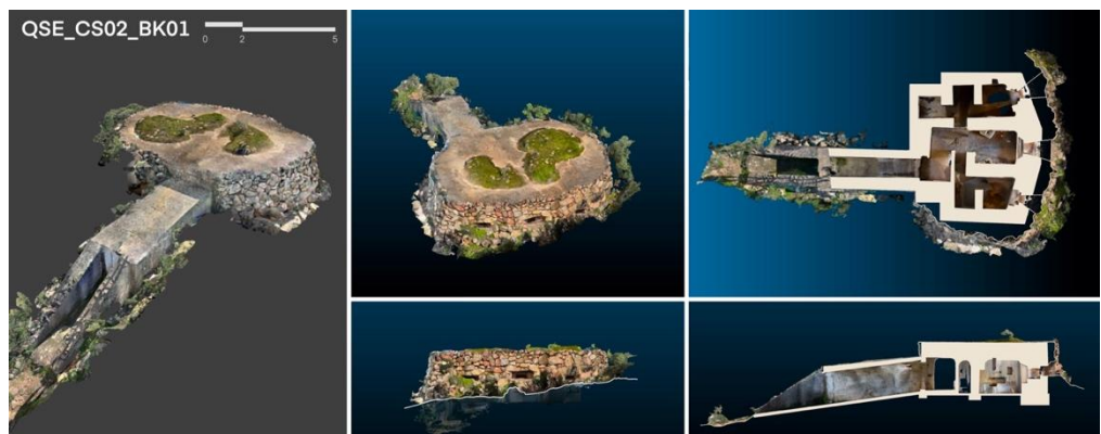
Fig. 7- Rilievo LiDAR: dal modello alla restituzione del BK01 (Restituzione grafica: G. Sanna)
