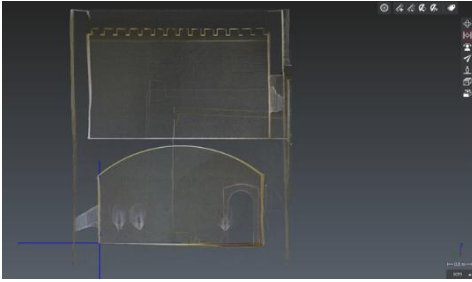
Fig. 17- Fase 2: Vista frontal (plano YZ) de la parte de la bóveda y muros de apoyo a estudio. (Autores)
