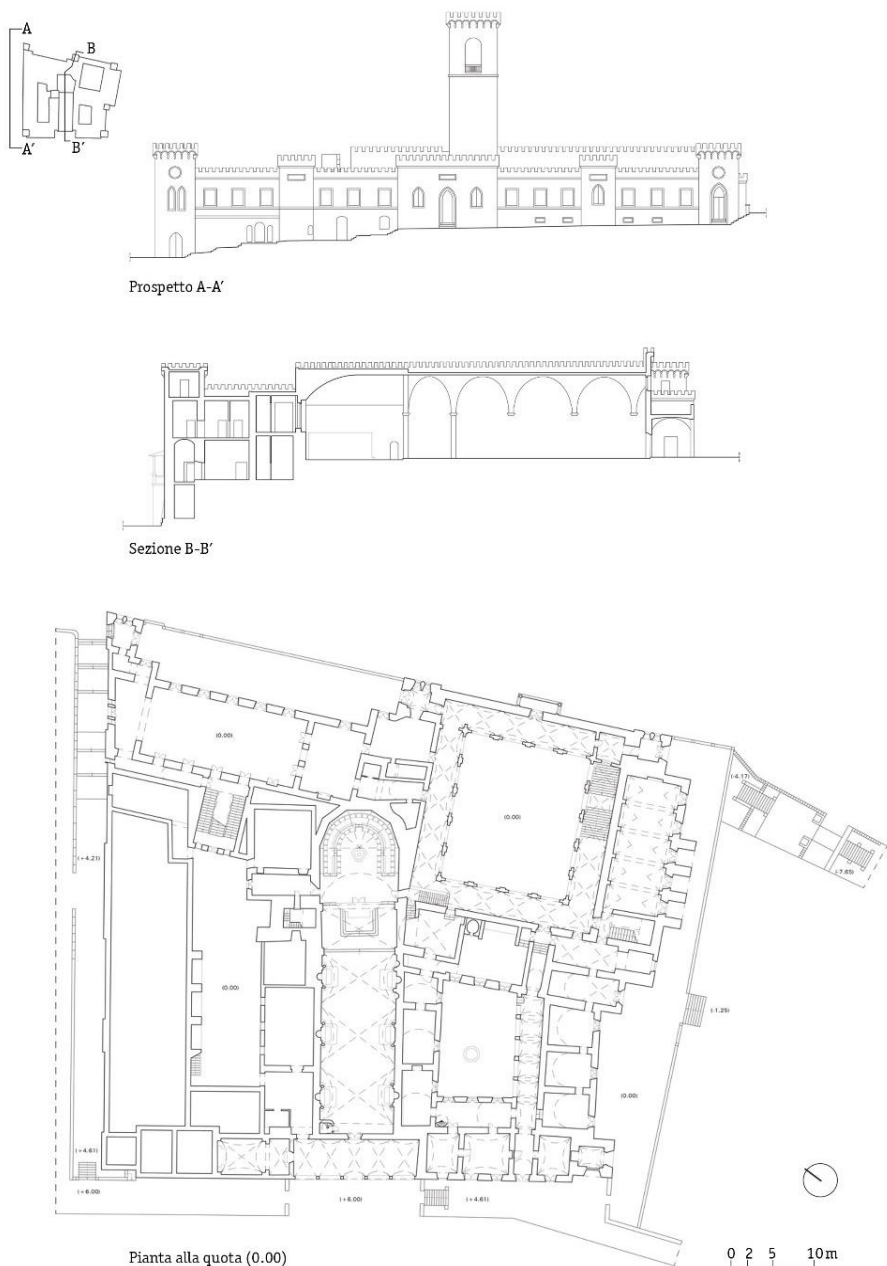
Fig. 4- Castello Guglielmi, ipotesi ricostruttiva, pianta, prospetto e sezione (elaborazione grafica di Chiara Spippoli, 2025)
