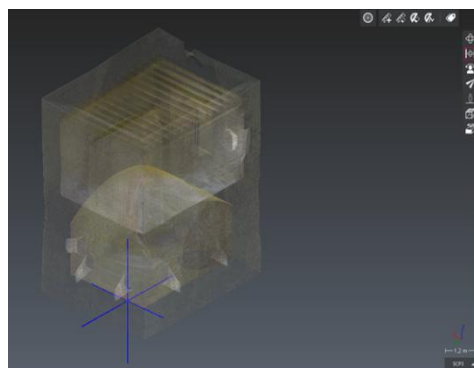
Fig. 16- Fase 1: nube de puntos parcial para el estudio de la bóveda de PBaja (torre suroeste). Ubicación del pto de ref.0.00. (Autores)
