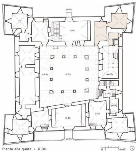
Fig. 7- Rilievo architettonico della Castellina a Norcia, pianta alla quota 0,00 m (elaborazione grafica di Serena Pallotti, 2025)
