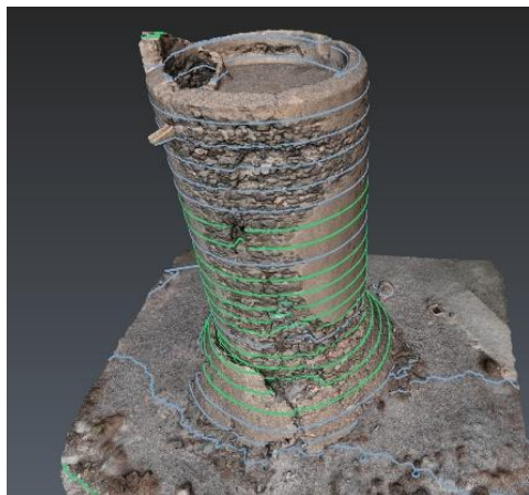
Fig. 7- Análisis geométrico de la torre Melicena mediante software Cyclone-3DShaper
