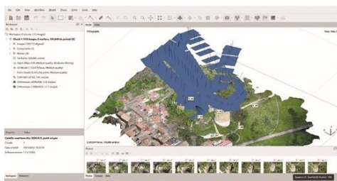
Fig. 6- Ambiente digitale SfM: prese di acquisizione del rilievo fotogrammetrico (elaborazione grafica di Domenico Iovane & Rosina Iaderosa, aprile 2025)
