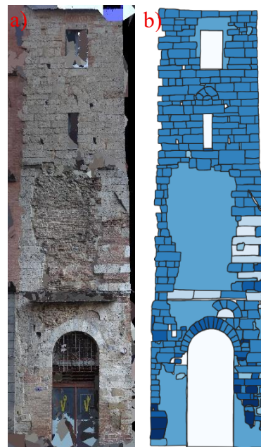
Fig. 5 a-b- a) Ortoproiezione della facciata Sud-Ovest della torre: b) mappatura litologica (elaborazione grafica degli autori, 2025)
