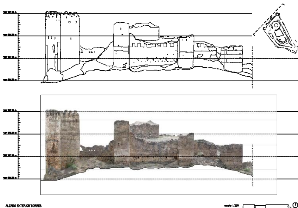
Fig. 7- Alzado exterior noroeste del castillo de Alcudia de Veo (elaboración gráfica por Ana Pérez-Vila, Teresa Gil-Piqueras & Pablo Rodríguez-Navarro, 2025)
