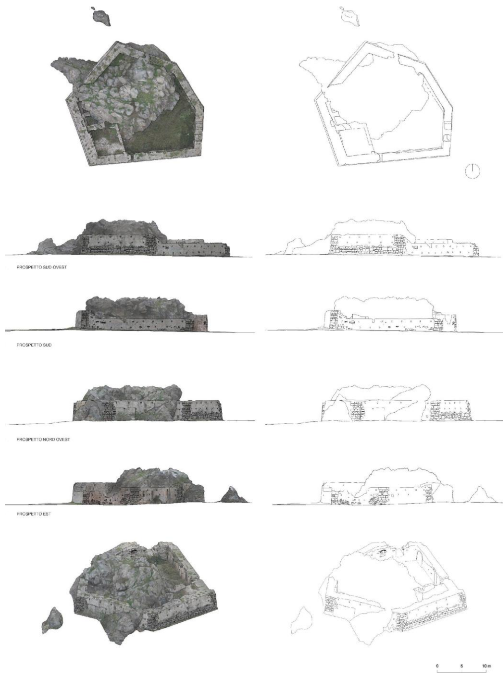
Fig. 5- Estratto degli elaborati di rilievo, pianta, prospetti e vista assonometrica (Acquisizione e restituzione L. Pizzonia)
