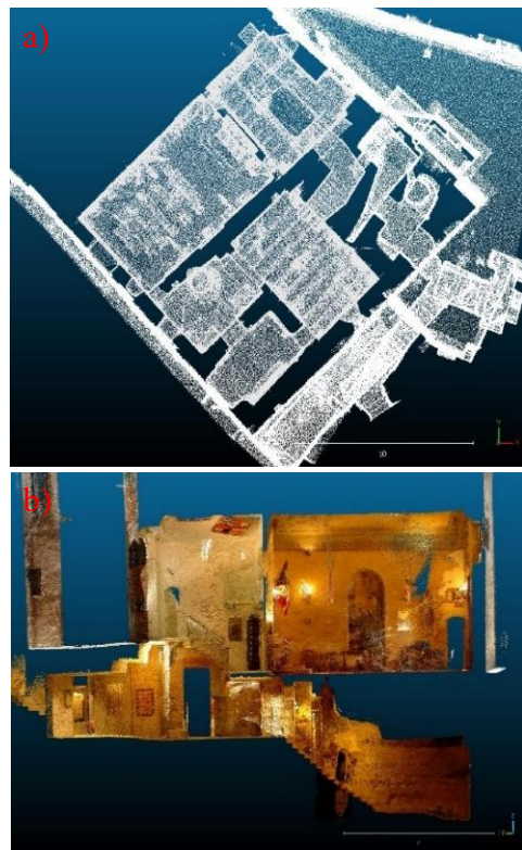
Fig. 6a-b- a) articolazione planimetrica di parte del palazzo Ugurgeri; b) sezione normale dove è possibile riconoscere ambienti di transito verticale, arredi e un ambiente ipogeo (elaborazione grafica degli autori, 2025)
