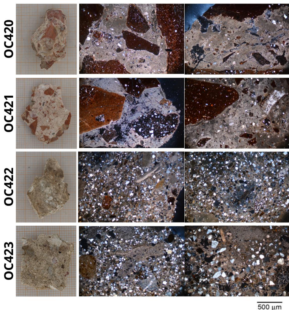
Fig. 7- Immagini di microscopia a luce polarizzata in sezione sottile di una selezione dei campioni di materiali analizzati (tutti ottenuti con nicols incrociati); OC420 e OC421 (blocchi in cocciopesto); OC422 e OC423 (malta dei blocchi di reimpiego in laterizio e malta) (elaborazione grafica degli autori, 2025)
