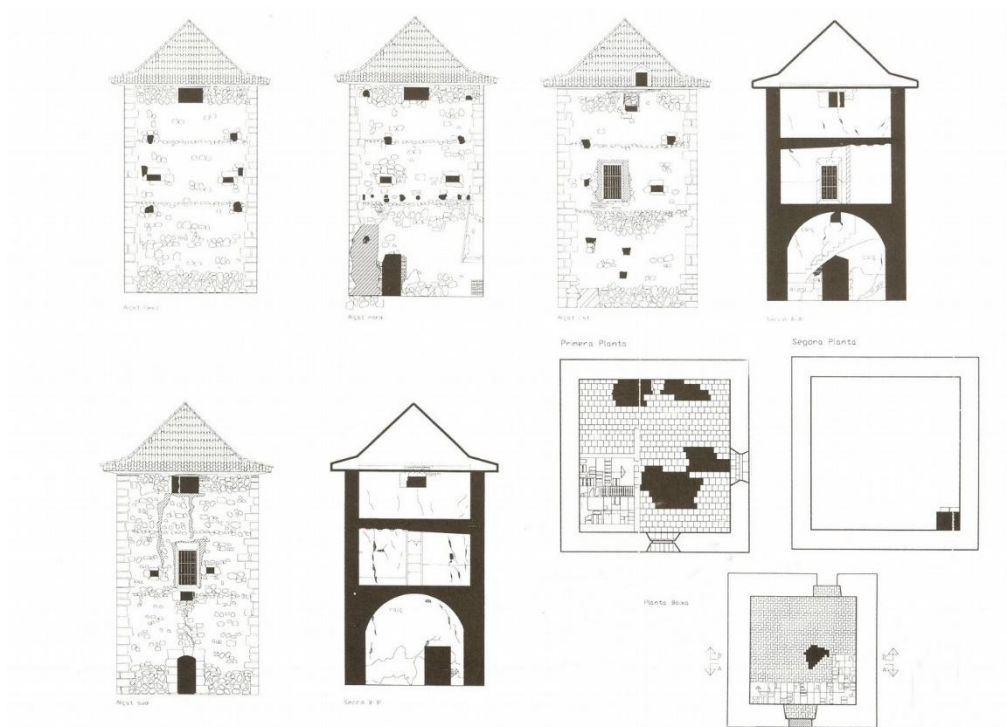
Fig. 8- Planimetría y alzado de la torre de Tadeo (Melchor, Benedito y Ferrer, 2001)
