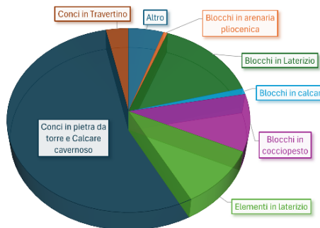
Fig. 6- Grafico a torta della composizione litologica della facciata Sud-Est (elaborazione grafica degli autori, 2025)
