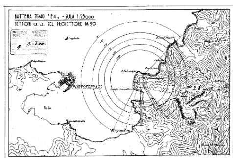
Fig. 6– Piano dei settori del proiettore da 90 della Batteria Costiera realizzata dalla Regia Marina tra il 1928 ed il 1933. (Fonte: archivio privato Giorgio Giusti)
