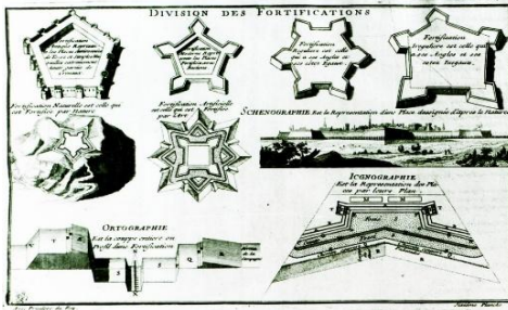
Fig. 3- Trattati e trattatisti; De Fer N., (1695). Introduction à la fortification par De Fer , Sixieme Planche, Division des Fortifications, (ed. Books Puddle, New York)
