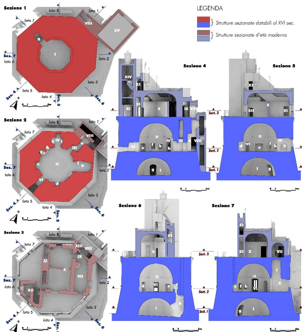
Fig. 4- Faro di Torre San Giovanni, Ugento (Le). Modello poligonale da rilievo laser scanner: sezioni
