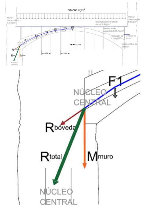
Fig. 25- Estudio y análisis de la estabilidad estructural mediante estática grafica a partir de la sección real obtenida a partir de la nube de puntos. (Autores)
