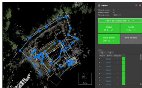
Fig. 14- Control de calidad del proceso de registro con error de cierre global de 1mm (Autores).
