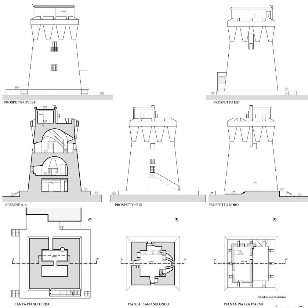
Fig. 9- Ricostruzione digitale bidimensionale della torre Vicereale di Lago Patria (CE) (elaborazione grafica di Michele Sabatino, 2025)
