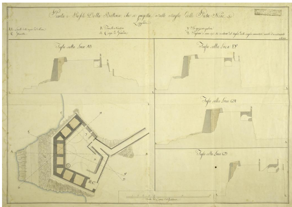
Fig. 3- Pianta e profili della batteria che si progetta sullo scoglio delle Pietre Nere (Colon. Montemajor, 1806-1815) (source: Biblioteca Nazionale di Napoli, sez. Manoscritti e rari, coll. CG b 25 b 64)
