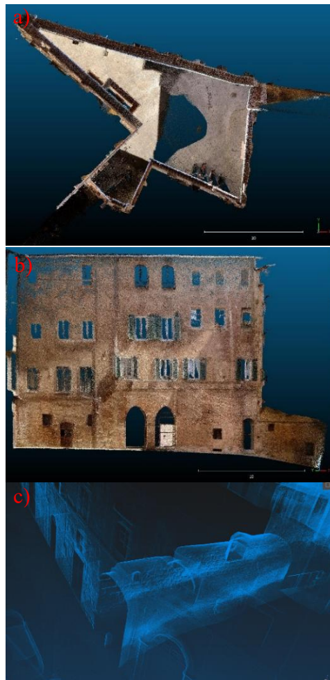
Fig. 5a-b-c- a) nuvola di punti vista dall'alto del cortile interno del Castellare; b) prospetto Nord-Est orto-corretto; c) particolare del vicolo voltato su via Cecco Angiolieri (elaborazione grafica degli autori, 2025)
