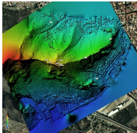
Fig. 11- Vista del MDE generado en el proceso fotogramétrico con Metashape Profesional de Agisoft (Autores)
