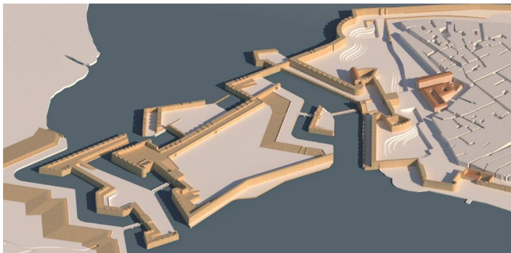
Fig. 9- Modello digitale raffigurante il sistema fortificato dell'istmo di Ortigia risalente al 1842. Vista da ovest (a cura dell'autrice)
